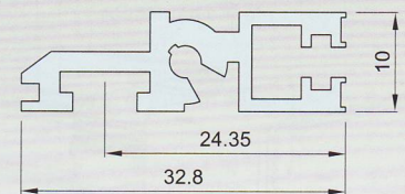
横梁(Beam)
