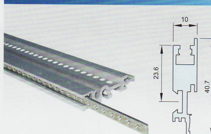
前横梁(Front beam)
