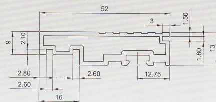
立柱(Vertical column)
