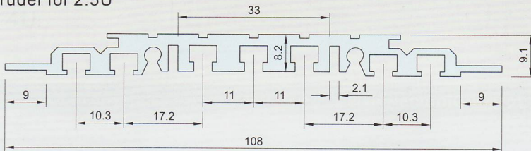
2.5U型材 Extruder for 2.5U
