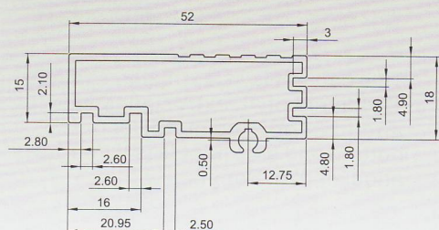
横梁(Beam)
