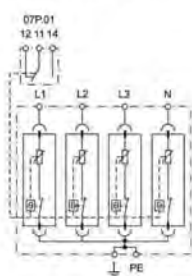
Схема № 7
