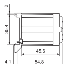
062.07 с реле
