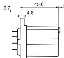
062.10 с реле
