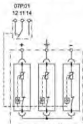
Схема № 14
