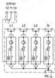
Схема № 13
