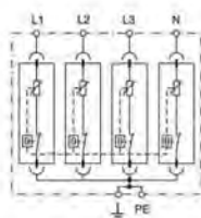
Схема № 8
