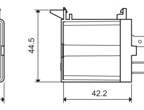
065.08 с реле
