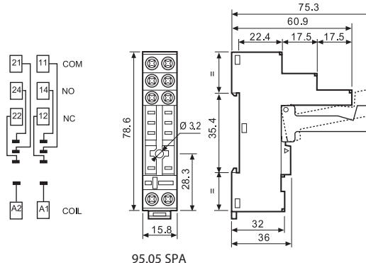
95.05 SPA
