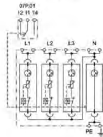
Схема № 12
