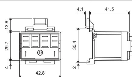
056.47 с реле
