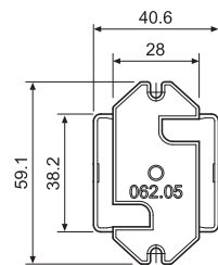
062.05
