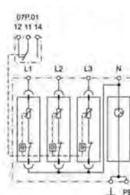
Схема № 5
