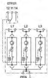
Схема № 11 bis
