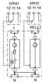
Схема № 11
