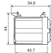
062.08 с реле
