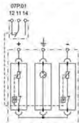
Схема № 13
