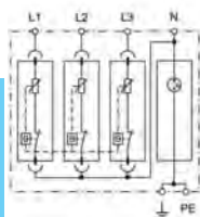
Схема № 6
