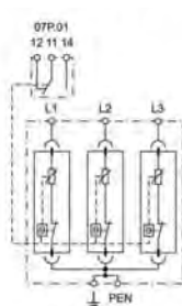
Схема № 4 bis
