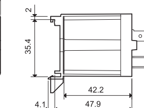
065.07 с реле
