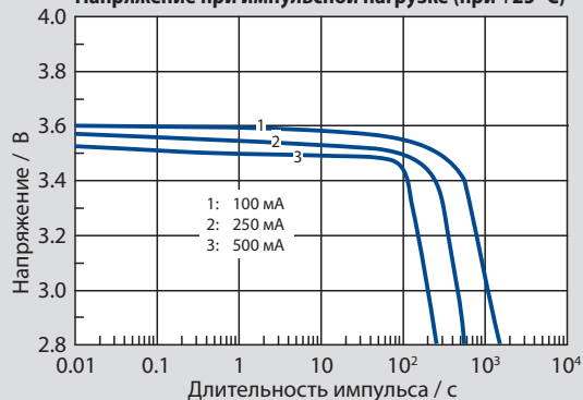
Напряжение при импульсной нагрузке (при +25 °C)
