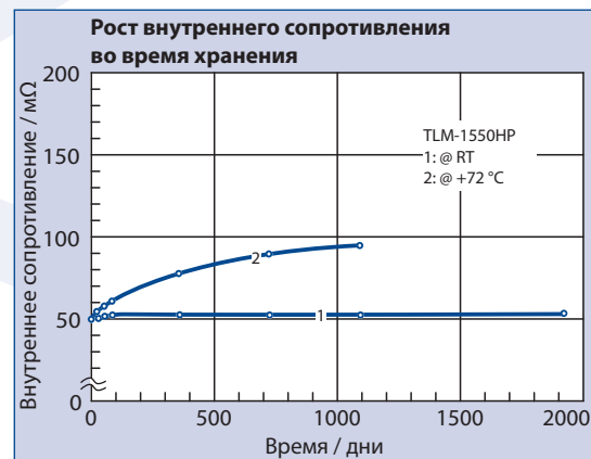
Рис. 3 Рост внутреннего сопротивления во время хранения
