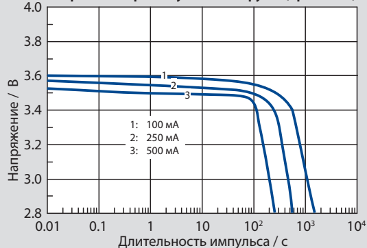
Напряжение при импульсной нагрузке (при +25 °C)
