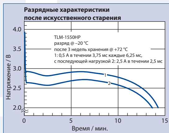
Рис. 2 Разрядные характеристики после искусственного старения
