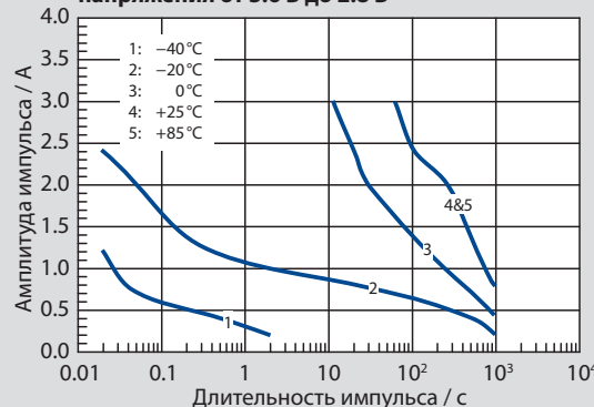
Напряжение в конце импульсной нагрузки длительностью 1 с
