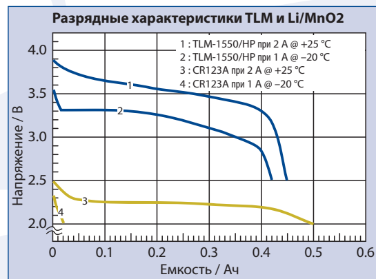
Рис. 1 Разрядные характеристики TLM и Li/MnO 2
