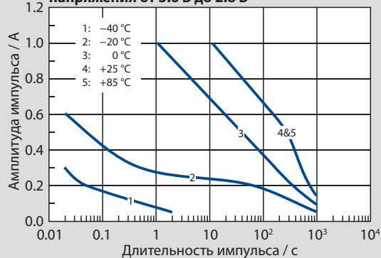
Напряжение в конце импульсной нагрузки длительностью 1 с
