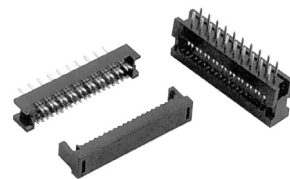
Вилка для наковки на плоский кабель с шагом 1.27 мм, открытая
