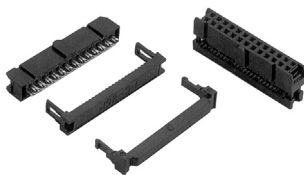
Розетка для наковки на плоский кабель с шагом 1.27 мм
