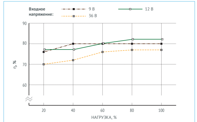
Рис. 4 (б). КПД VDN10B05.
