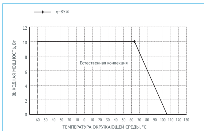
Рис. 6. Тепловая кривая VDN10.
