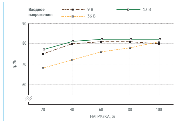
Рис. 4 (г). КПД VDN10B12.
