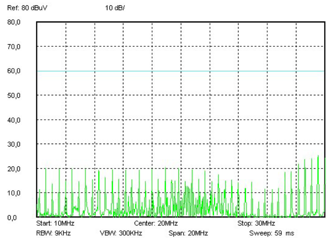
Рис. 10 (б). Спектрограмма 10–30 МГц.
