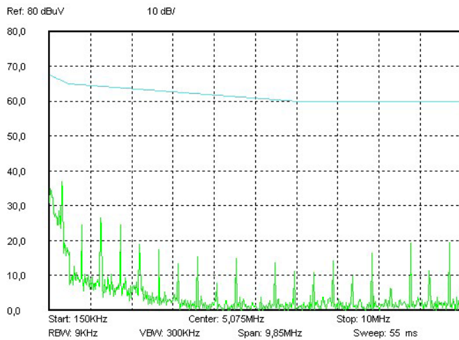
Рис. 10 (а). Спектрограмма 0,15–10 МГц.
