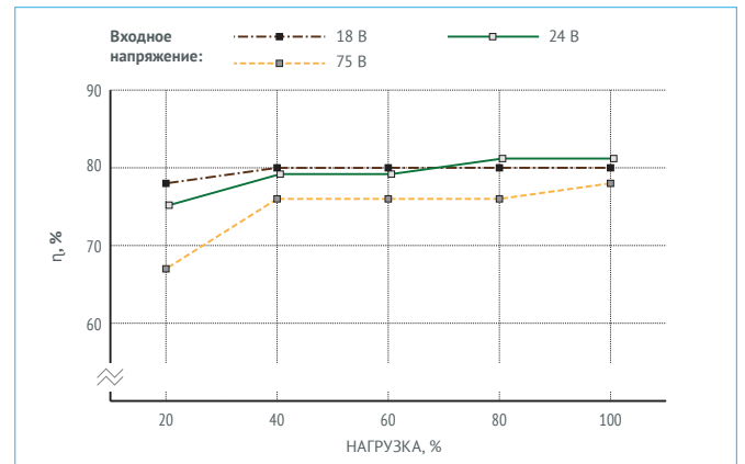
Рис. 5 (б). КПД VDN10W05.
