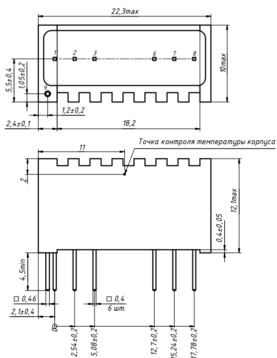
Рис. 11. Стандартное исполнение VDN10.
