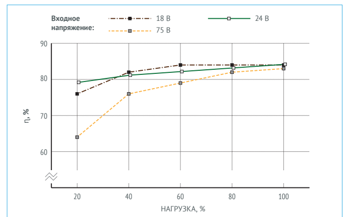
Рис. 5 (г). КПД VDN10W12.
