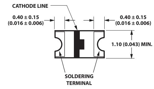
HSMx-C177
