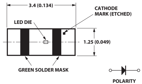
HSMx-C177
