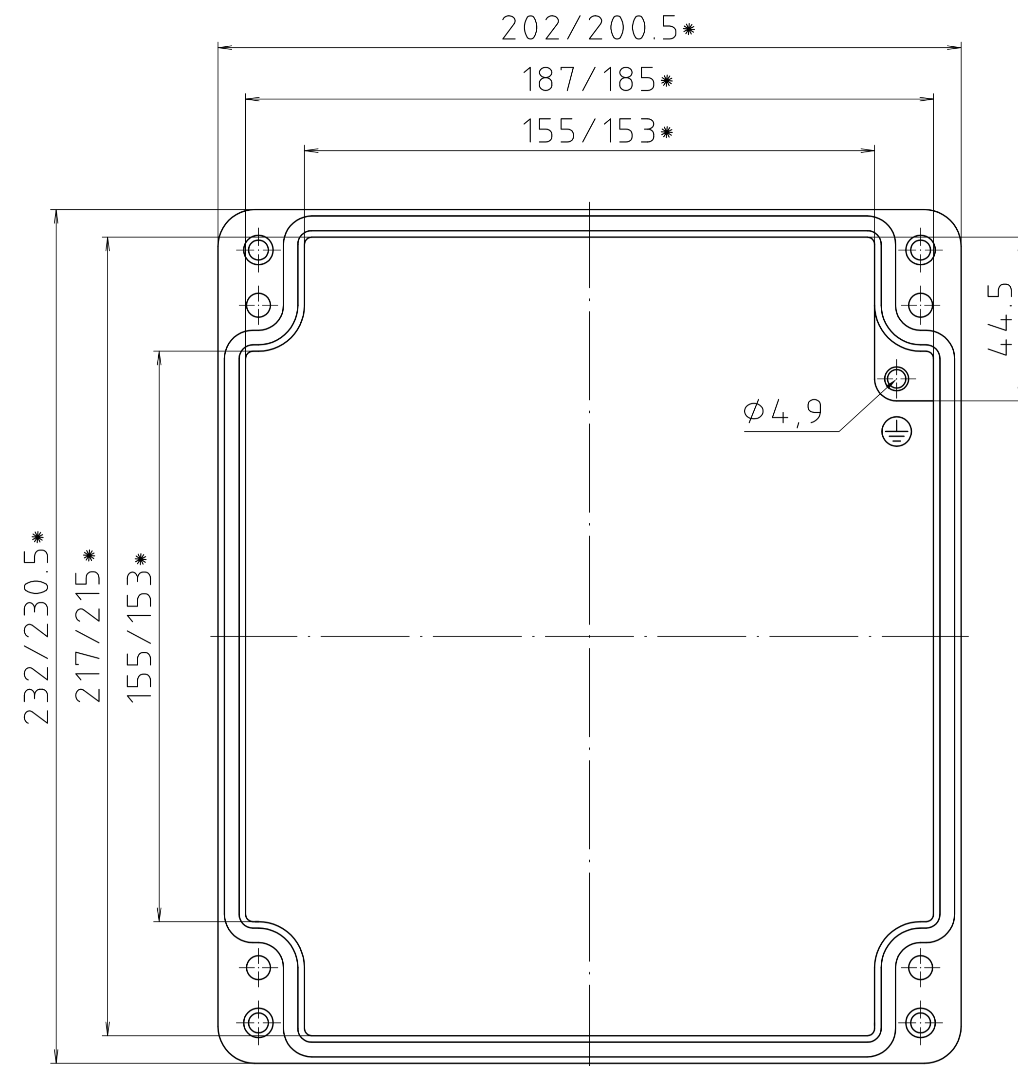
Deckel / lid
