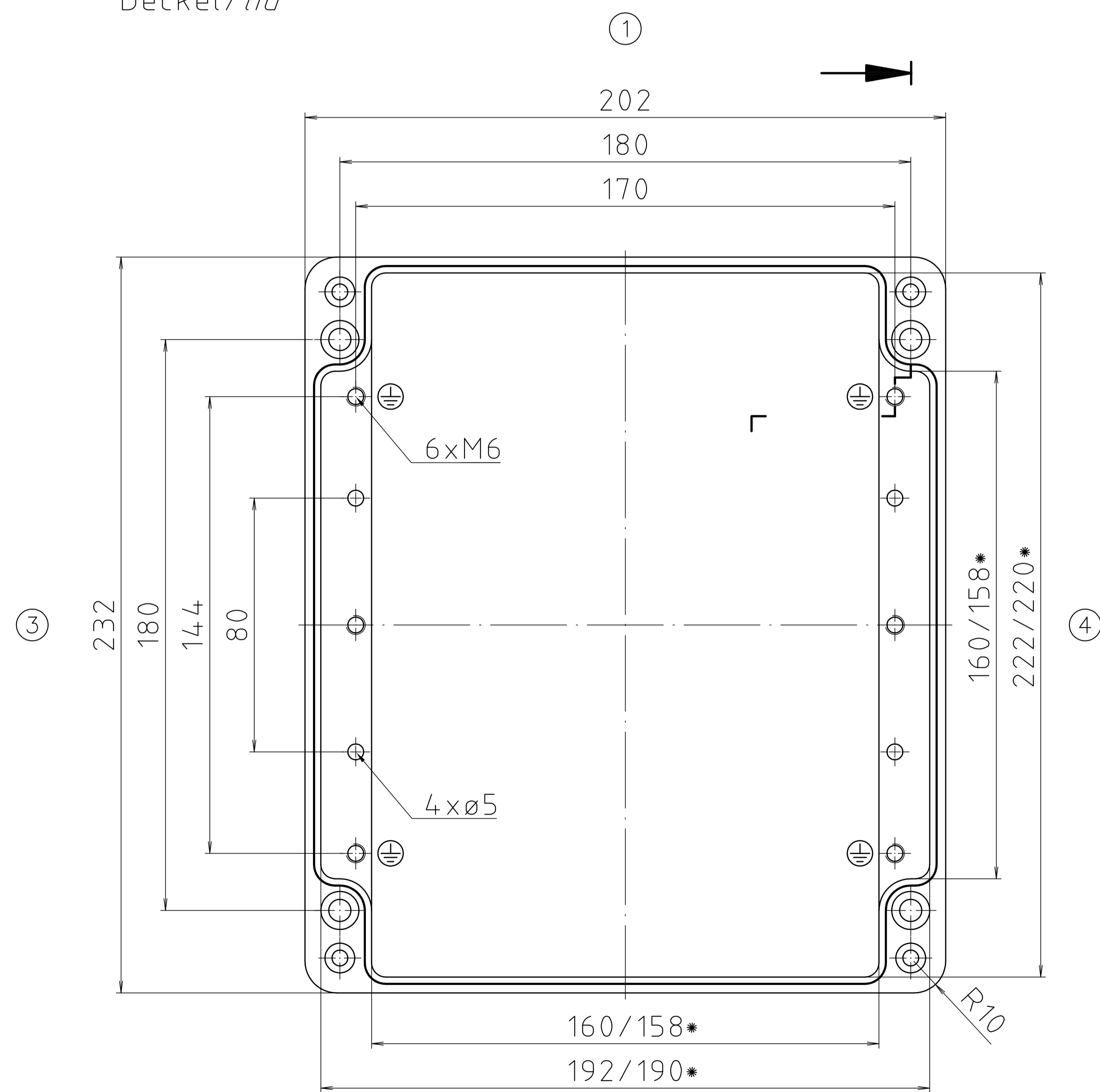
Unterteil / base
