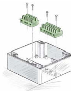
Упоры для клеммных колодок, например, (тип KL 16, фирмы Wieland).
