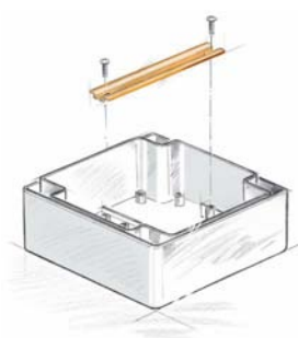
Упоры с боковыми рёбрами для устойчивого монтажа несущей шины
