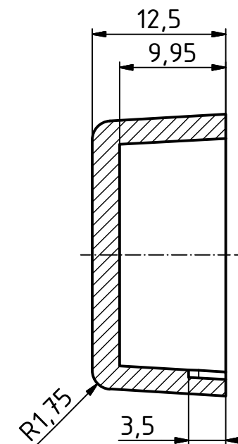
C-C ( 2 : 1 )
