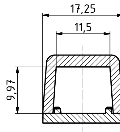
A-A ( 2 : 1 )
