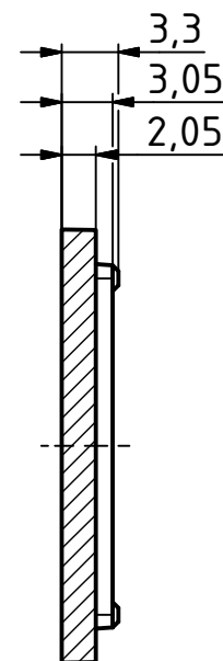
B-B ( 2 : 1 )
