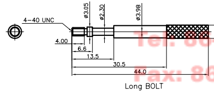
Long BOLT
