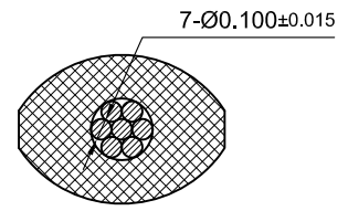
SECTION A-A (4:1)
