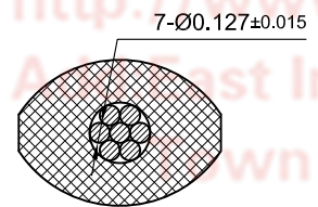
SECTION A-A (4:1)
