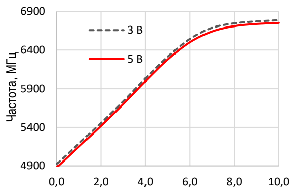
ДИАПАЗОН ПЕРЕСТРОЙКИ
