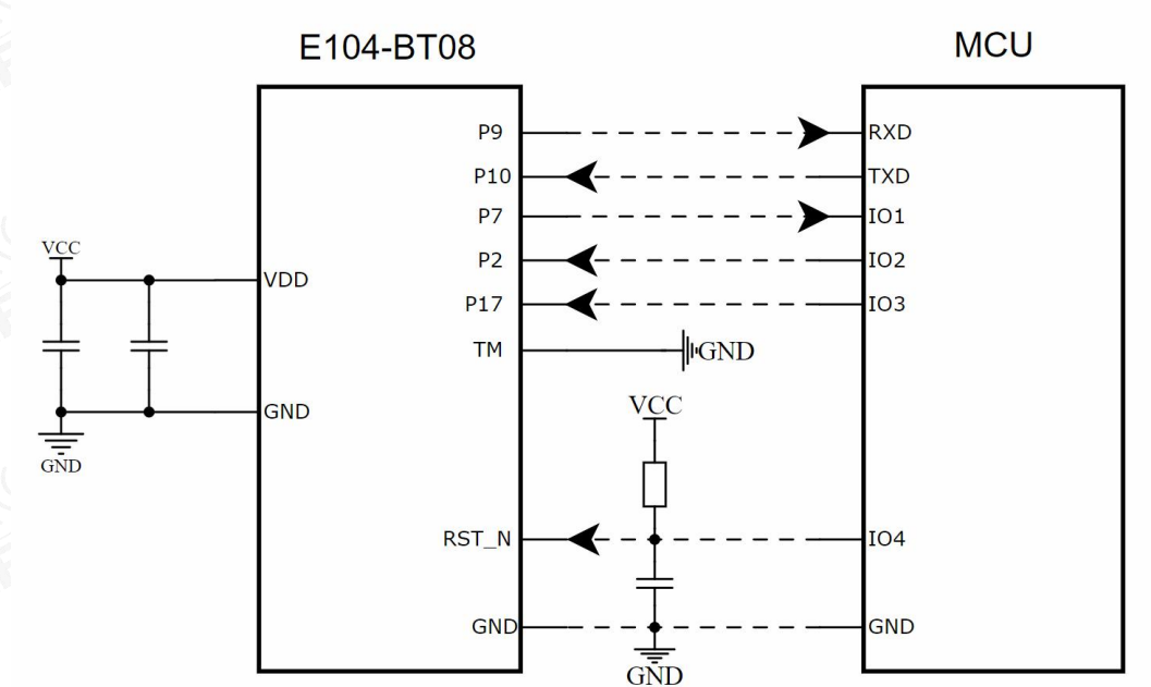
Figure 4-2 E104-BT08 Circuit
