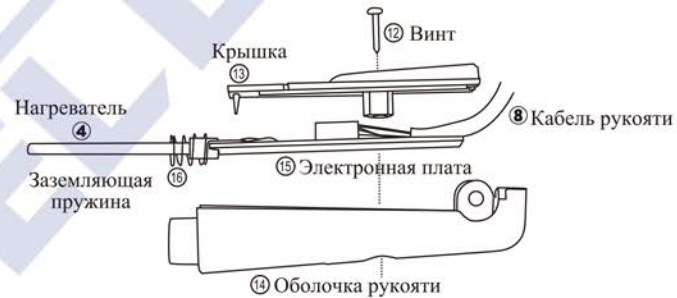
Рис. 4 Замена нагревателя
