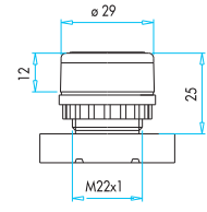
Düz, Yaylı Flush
