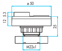
Çiftli Çıkık Kafalı, Yaylı Double Extended, Spring Return
