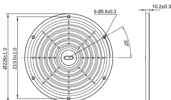
FPG-20 для 200 мм вентилятора
