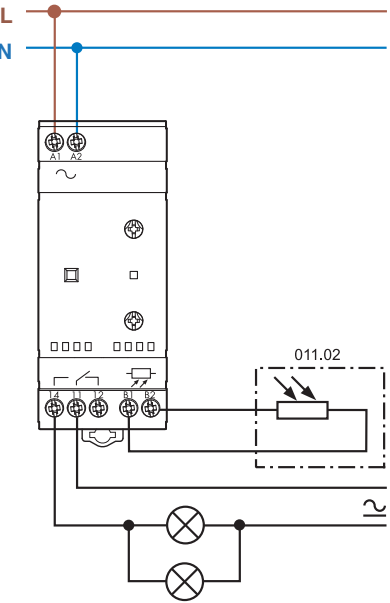
Тип 11.91 + 19.91
