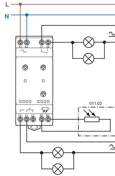
Тип 11.42
