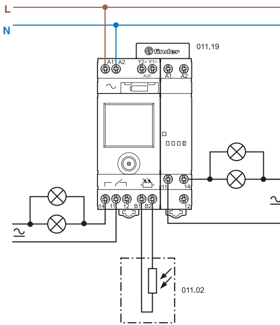
Тип 11.91 + 19.91
