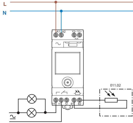
Тип 11.91
