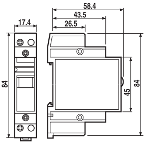
Тип 22.23 Винтовой зажим
