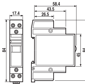
Тип 22.24 Винтовой зажим
