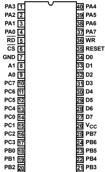
82C55 (PDIP, Cerdip)
