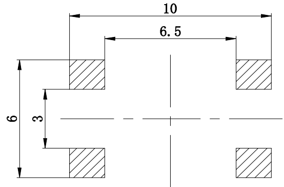
安装尺寸
