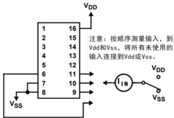
Fig.4 输入电流
