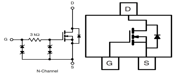
SOT-23
