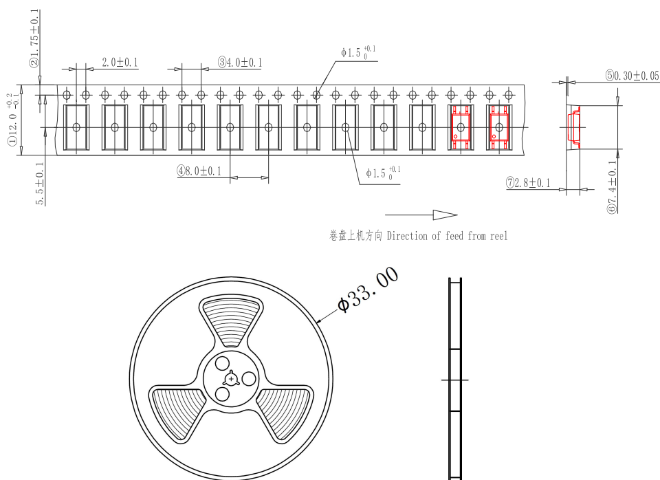
图 13 编带包装示意图
