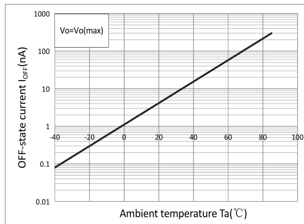
图 6 I OFF -T a 特性曲线
