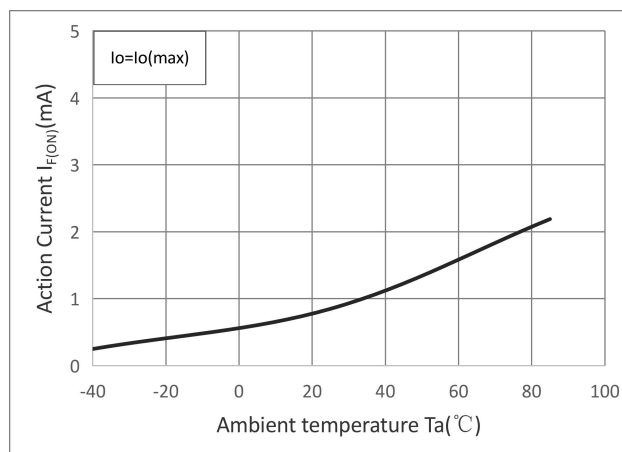
图 8 I F(ON) -T a 特性曲线
