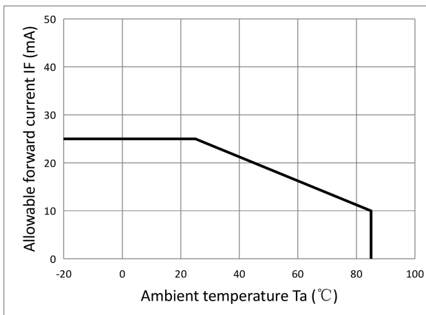
图 3 I_F - T_a 特性曲线
