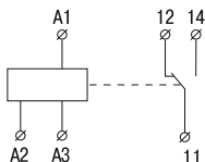
Рисунок A.1 – Схема подключения OIR-116 Figure A.1 – OIR-116 wiring diagram
