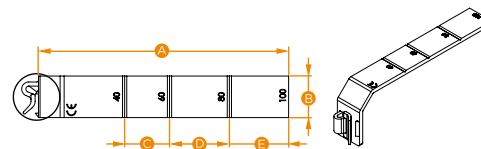
Разделитель уровней
