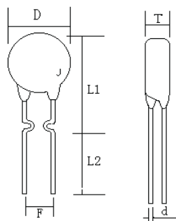
Long internal curvature 长内弯 侧面 Side
