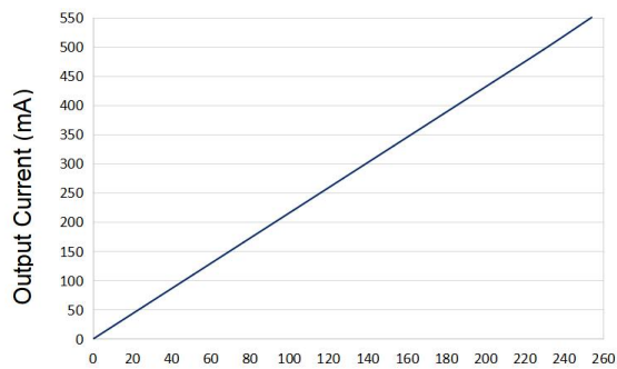
Linear dimming
