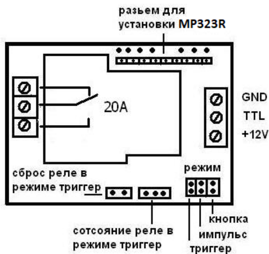
Схема подключения
