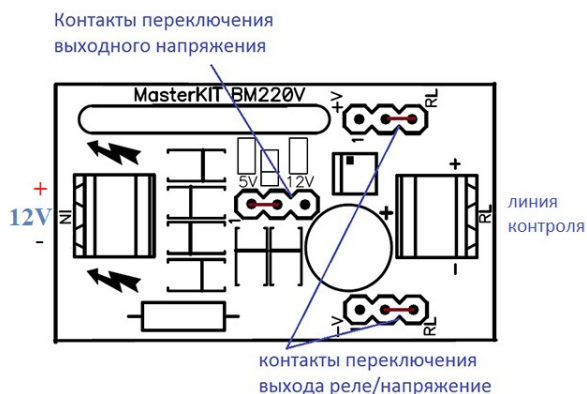
Эскиз подключения
