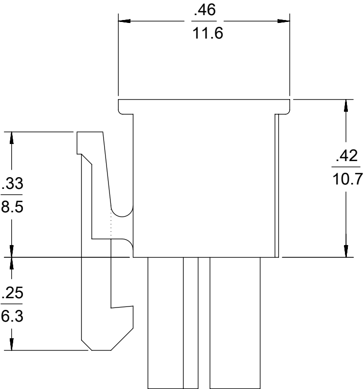
4-24 CKT
