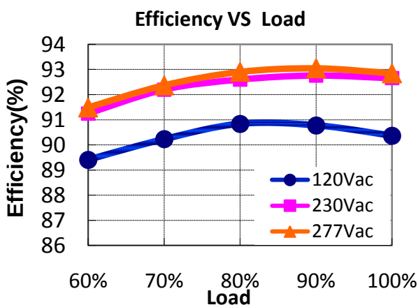
MTP-200X068( I_o=2.95A )
