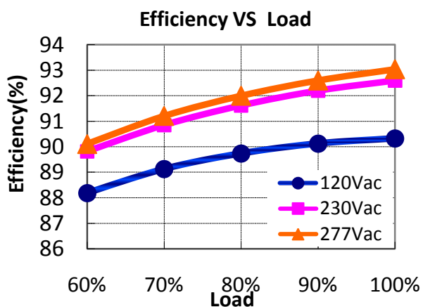
MTP-200X068( I_o=3.60A )
