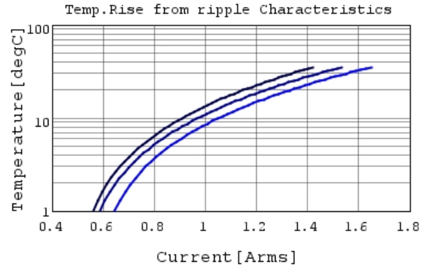
GQM2195C2E300GB12 Temp.rise 500MHz
