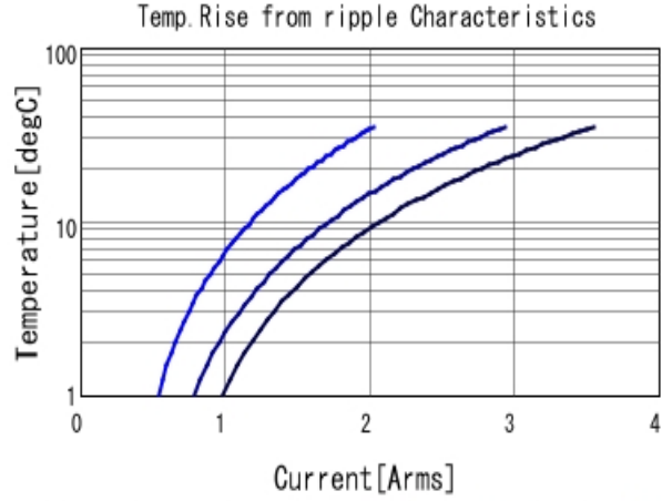
GRM31MR71H474KA01 Temp. rise ■ 200kHz ■ 500kHz ■ 1MHz
