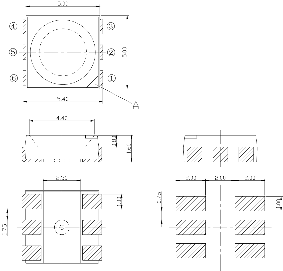
推荐焊盘
