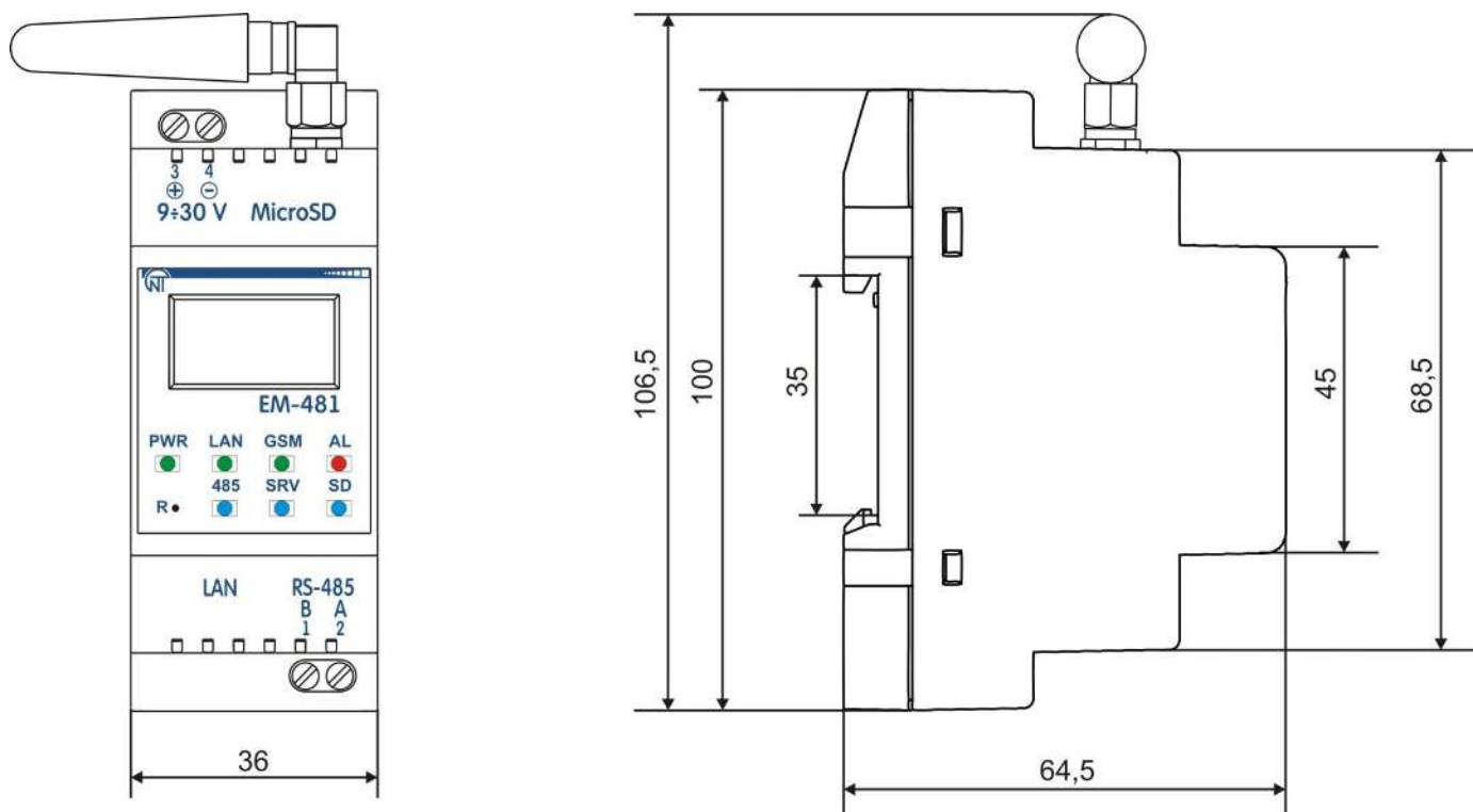
Рисунок 1.1 – Габаритные и установочные размеры EM-481
