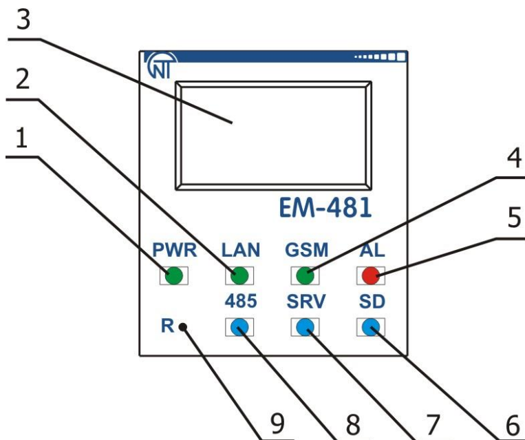
Рисунок 1.2 – Органы управления EM-481
