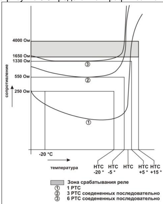
Рисунок 5.3 – График зависимости сопротивления датчика РТС от температуры
