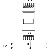
Схема подключения
