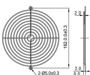
FG-15 для 150 мм вентилятора
