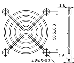
FG-06 для 60 мм вентилятора
