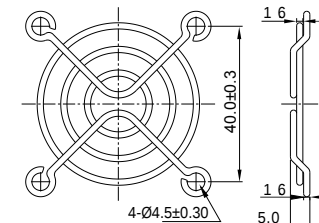
FG-05 для 50 мм вентилятора
