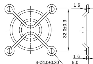
FG-04 для 40 мм вентилятора
