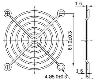
FG-07 для 70 мм вентилятора
