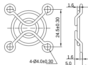
FG-03 для 30 мм вентилятора
