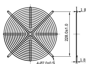
FG-25 для 250 мм вентилятора
