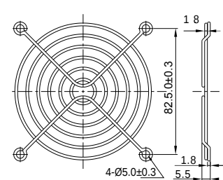
FG-09 для 90 мм вентилятора
