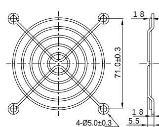
FG-08 для 80 мм вентилятора
