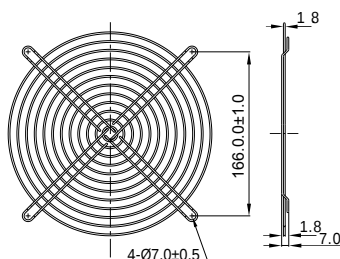
FG-20 для 200 мм вентилятора
