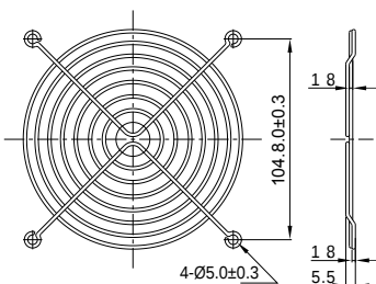
FG-12 для 120 мм вентилятора
