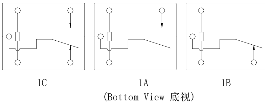
Wiring Diagram 接线图
