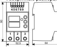
Габаритные размеры
