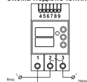
Схема подключения
