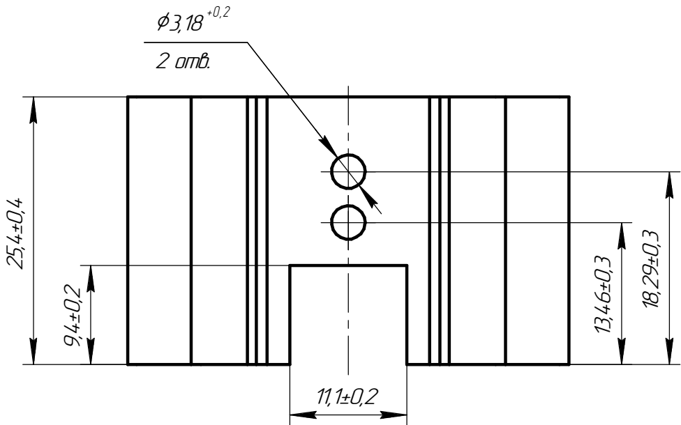
Исполнение ABM 2000.04.444_ФАП.8511-01
