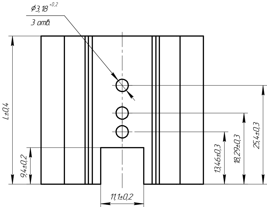
Исполнение ABM 2000.04.444_ФАП.8511-02, -03, -04
