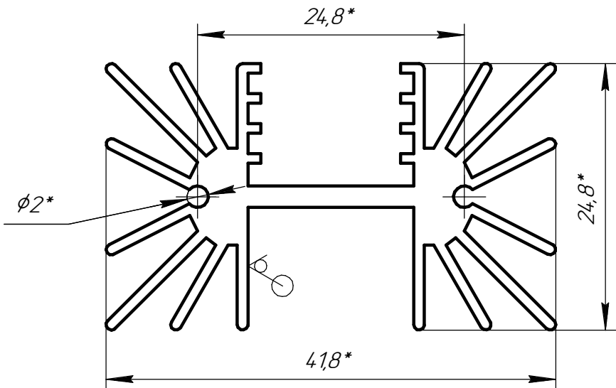
Исполнение ABM 2000.04.444_ФАП.8511-01
