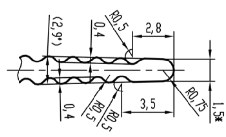
A(4:1) 18 мест
