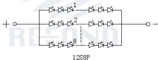
Fig.1-3 Polarity 极性
