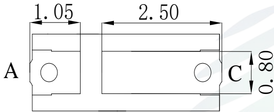
Fig. 1-3 Bottom View 背面视图
