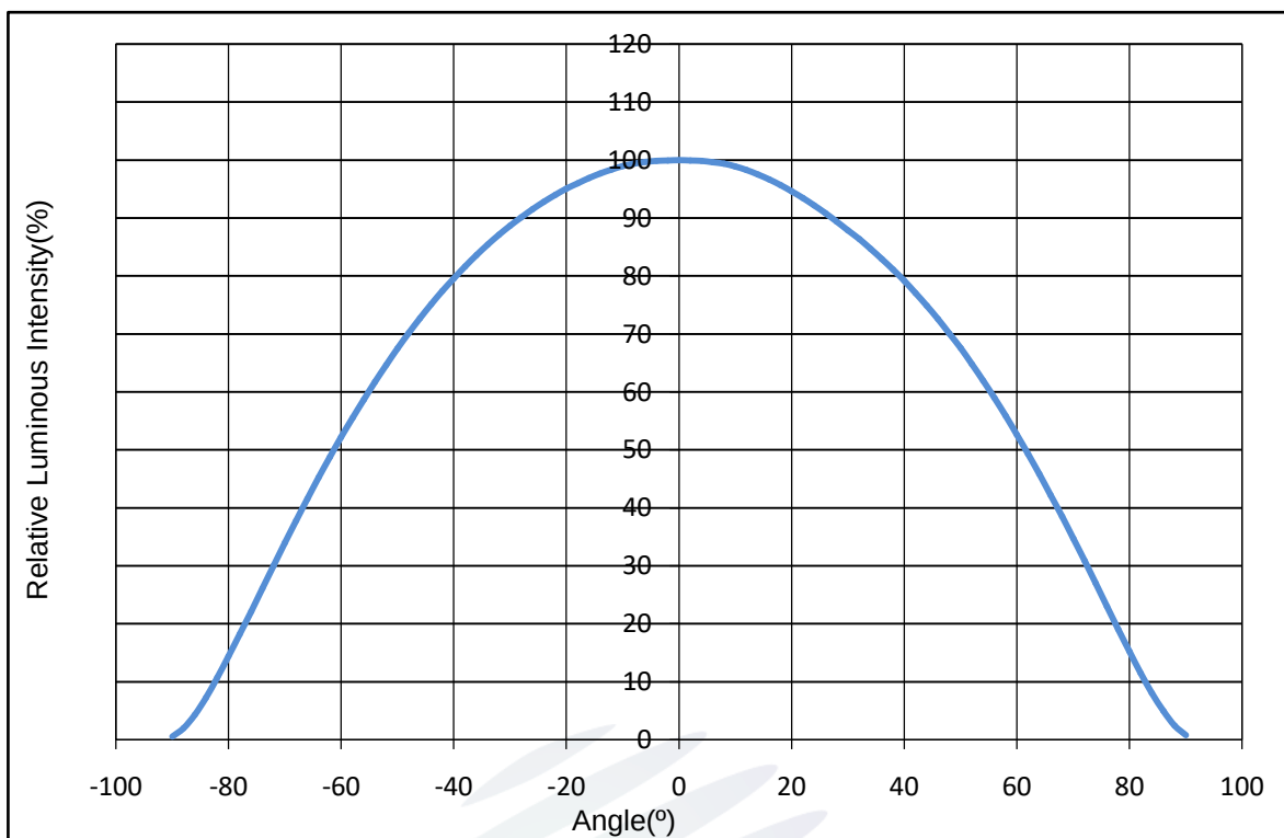
Fig. 1-13 Radiation diagram 辐射特性曲线
