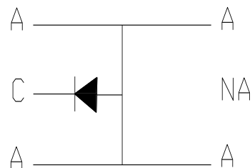
Fig.1-4 Polarity 极性
