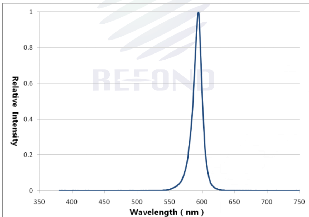
Fig. 1-14 Spectrum Distribution 光谱分布特性曲线
