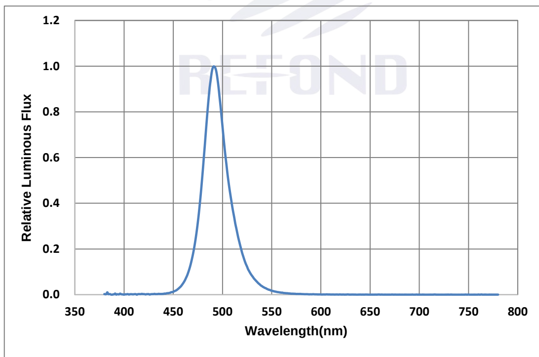
Fig. 1-16 Spectrum Distribution 光谱分布特性曲线
