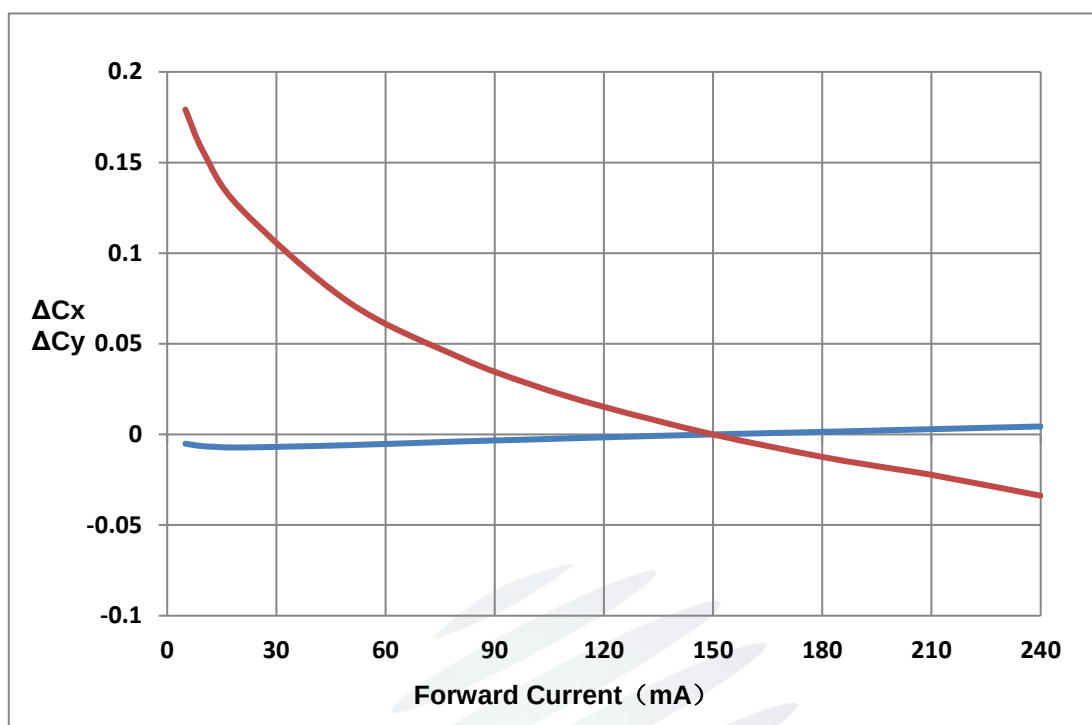
Fig. 1-15 Chromaticity Coordinate Shift Vs Forward Current 色坐标偏移与正向电流特性曲线
