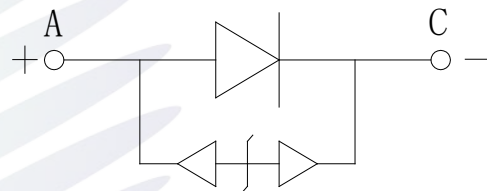
Fig.1-4 Polarity 极性
