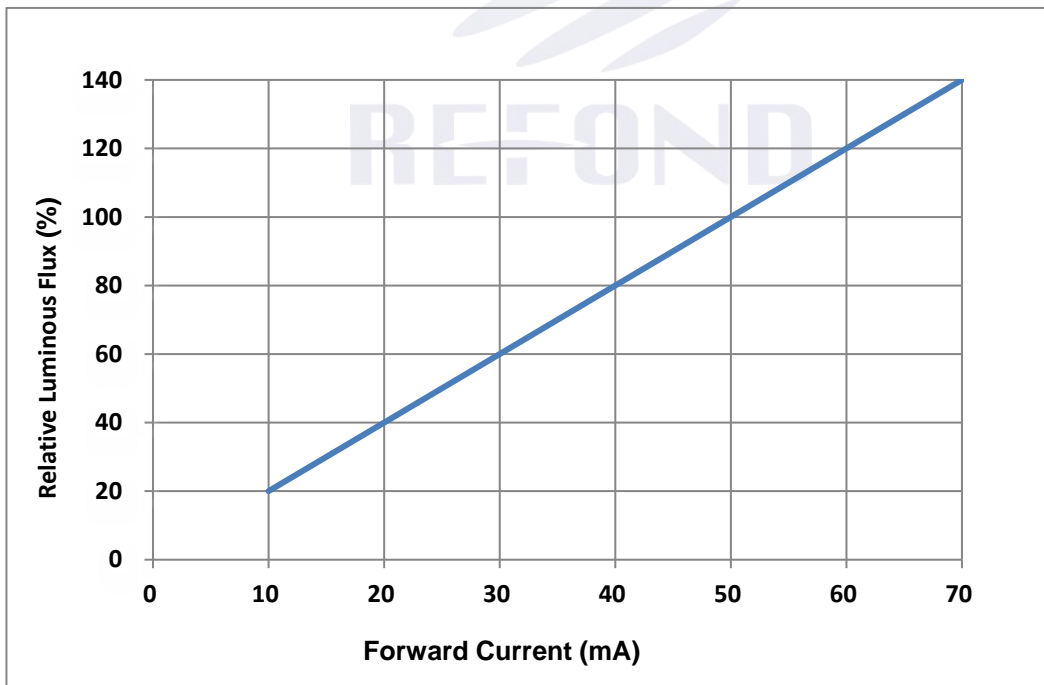
Fig. 1-8 Forward Current Vs Relative flux正向电流与相对光通量特性曲线
