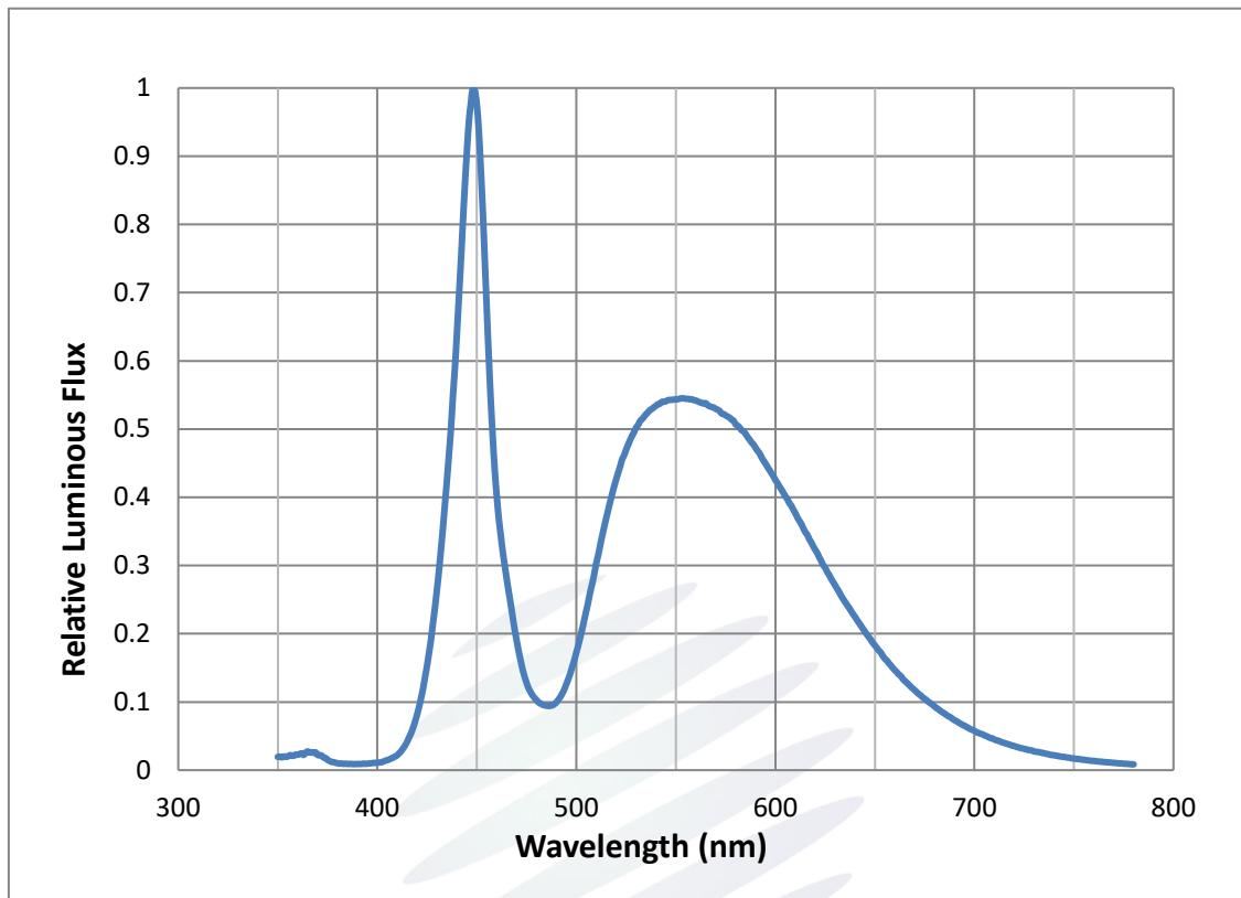
Fig 1-15 Spectrum Distribution 光谱分布特性曲线
