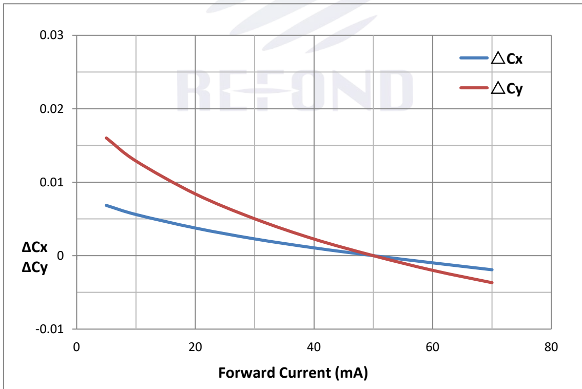
Fig.1-14 Forward Current vs. Color Shift 正向电流与色坐标偏移特性曲线
