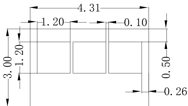
Fig.1-1 Top View 正面视图
