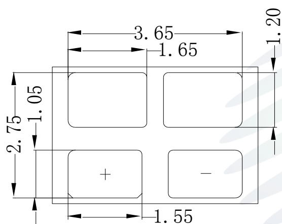
Fig.1-3 Bottom View 背面视图
