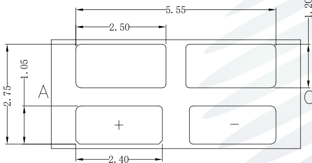
Fig.1-3 Bottom View 背面视图
