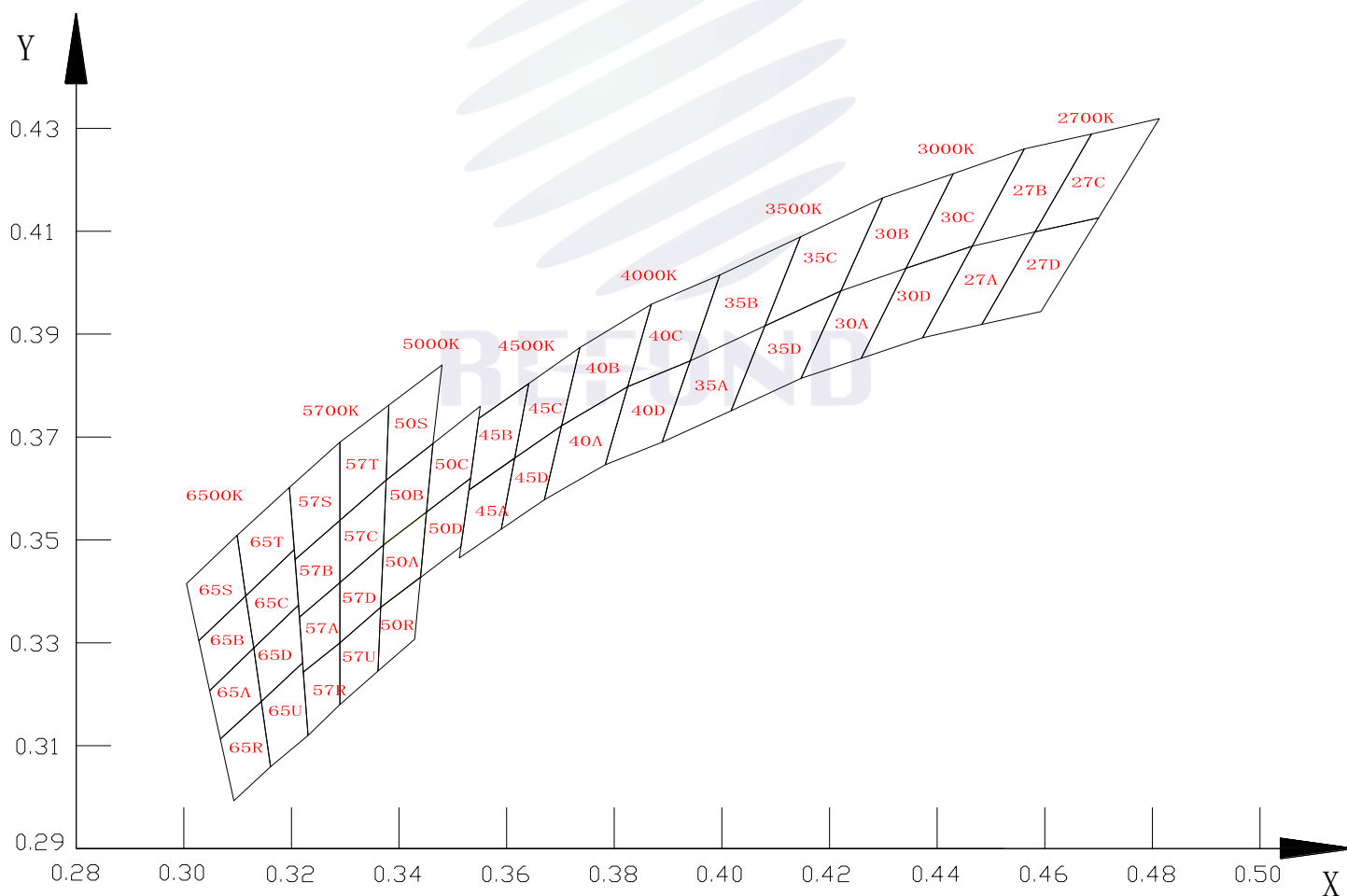
Fig.1-7 Chromaticity Coordinates 正向电流与相对光强特性曲线 Table 1-4 Chromaticity Region & Coordinates
